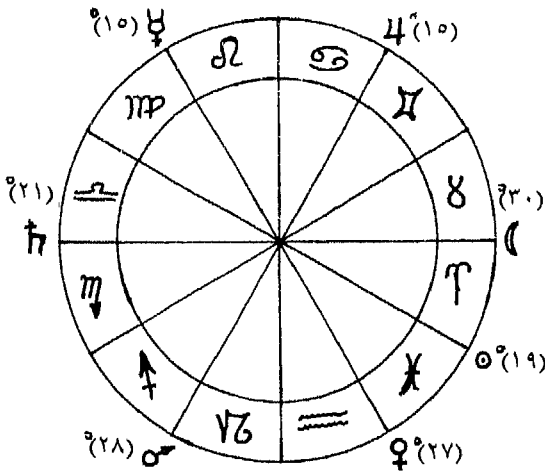
شكل (١٦) : أماكن إشراف وهبوط الكواكب
